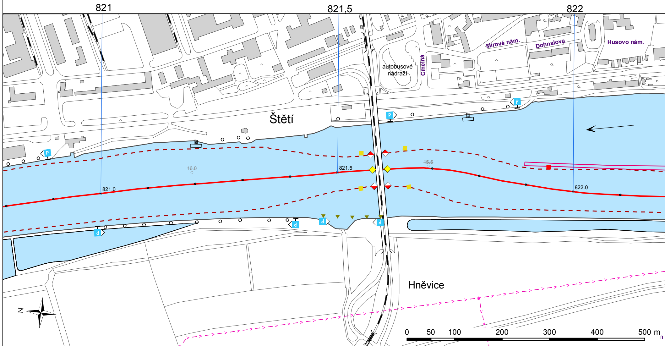
821,59 Štětí, silniční a železniční most, podjezdová výška k max. vodnímu stavu 5,66 m Most 15
